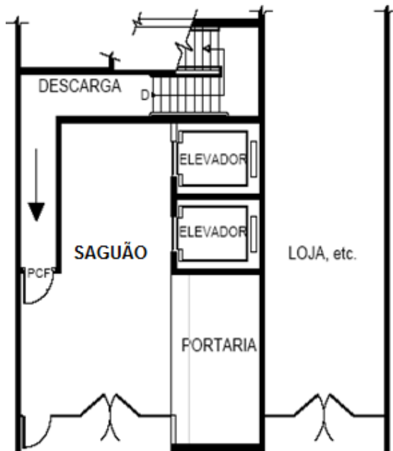
Figura 23 – Descarga através de hall térreo enclausurado
