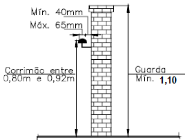
Figura 19 – Dimensões de guardas e corrimãos
